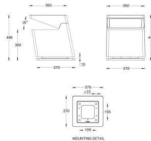
FRAME FRA-10001
