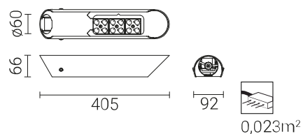
ISKRA LED P PROG na przejścia dla pieszych dla dróg z ruchem lewostronnym
