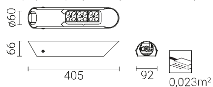
ISKRA LED P PROG na przejścia dla pieszych dla dróg z ruchem lewostronnym
