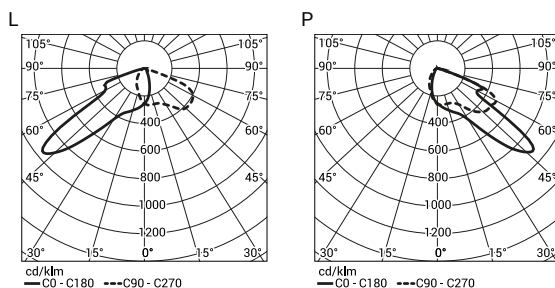
ISKRA LED P PROG na przejścia dla pieszych dla dróg z ruchem lewostronnym
